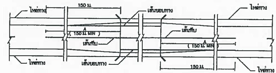
การเว้นระยะของช่องจราจรที่ความกว้างจราจรถนน
