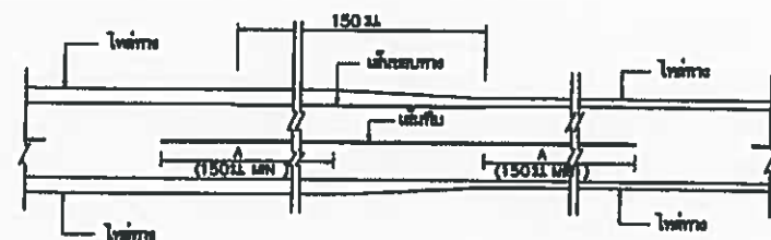
การตั้งเส้นจราจร การเว้นระยะของไหล่ทางตรง
