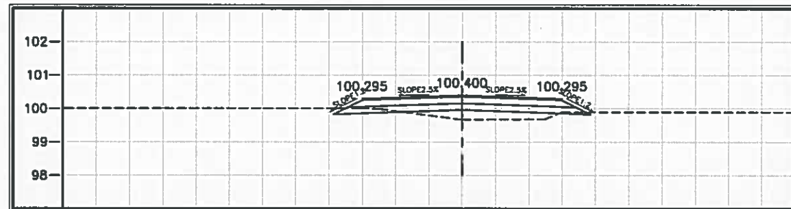
STA. 1+875.000 NGL = 99.670
