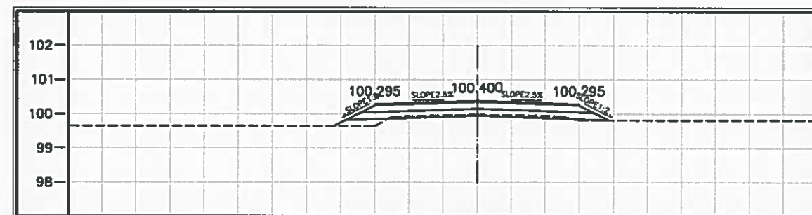
STA. 1+925.000 NGL = 99.985
