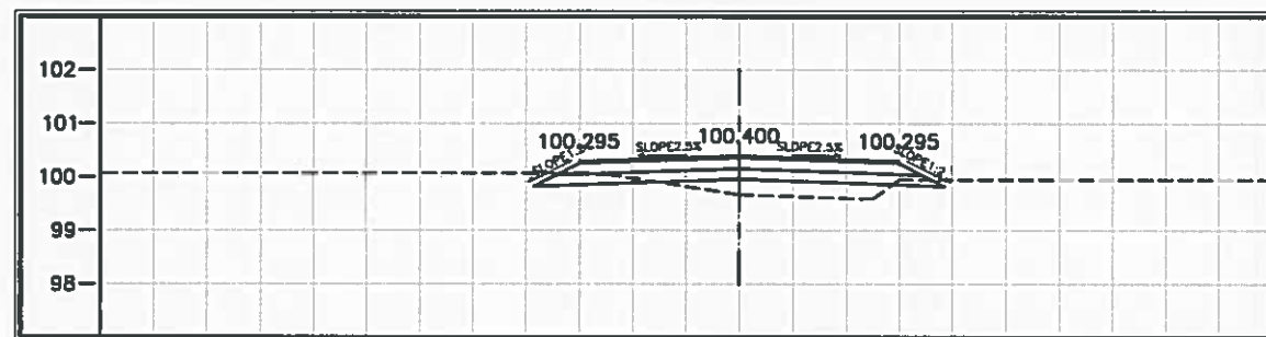
STA. 1+850.000 NGL = 99.670
