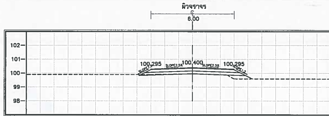
STA. 1+900.000 NGL = 99.950
