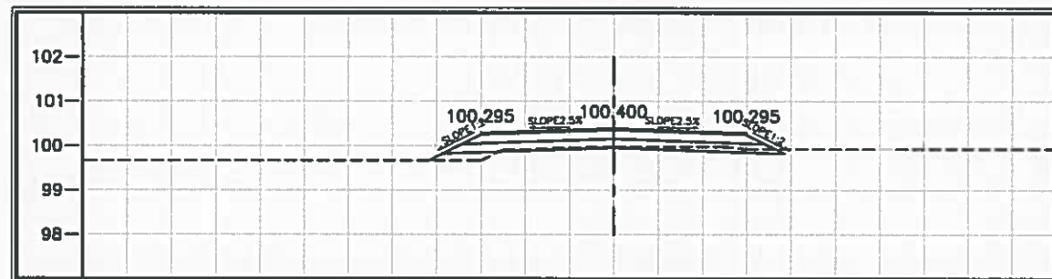
STA. 1+825.000 NGL = 99.980
