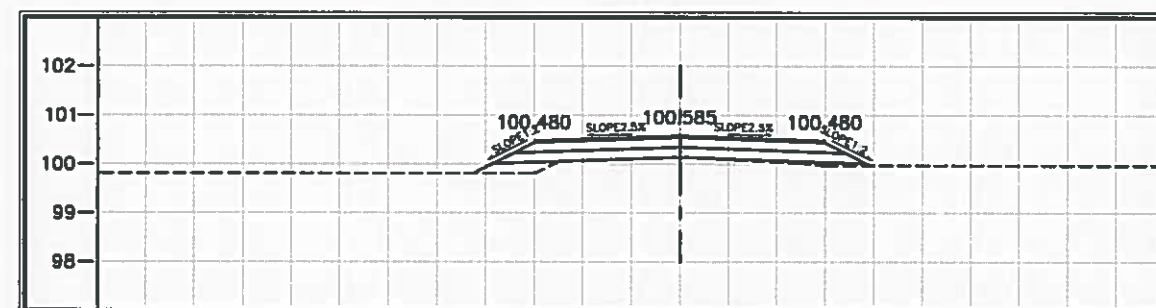
STA. 1+950.000 NGL = 100.140
