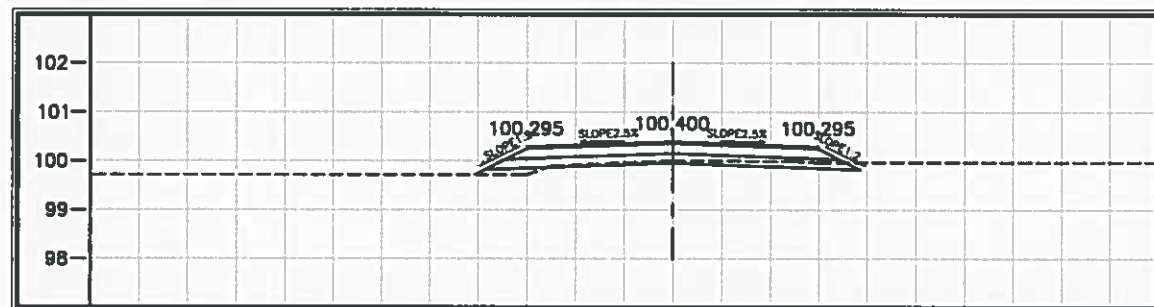
STA. 1+800.000 NGL = 100.010
