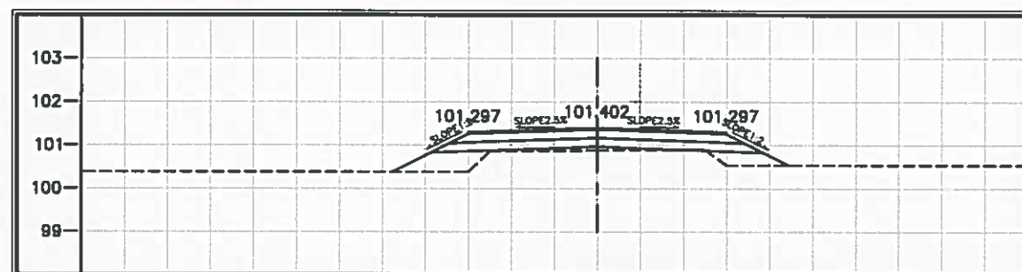
STA. 2+475.000 NGL = 100.877
