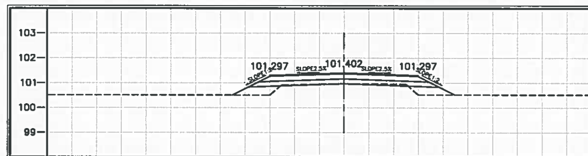
STA. 2+500.000 NGL = 100.967
