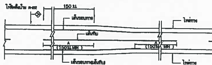
การตั้งเส้นจราจร การเว้นระยะของช่องจราจรตรง
