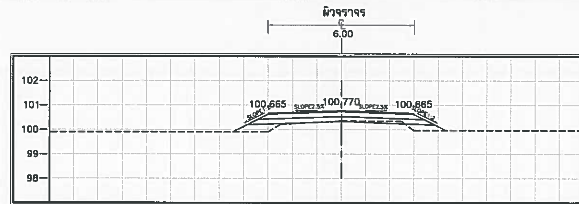
STA. 2+000.000 NGL = 100.380
