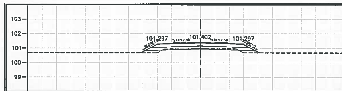
STA. 2+550.000 NGL = 100.962
