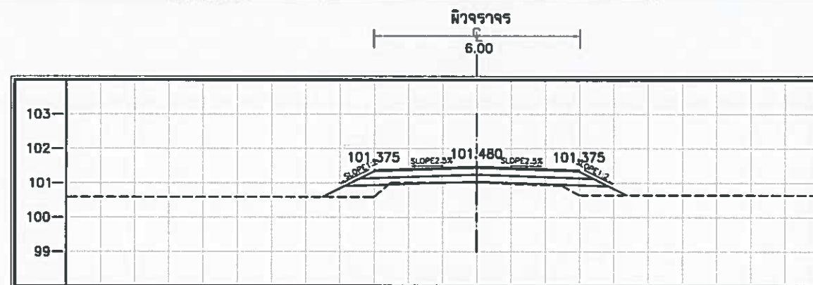
STA. 2+575.000 NGL = 101.012
