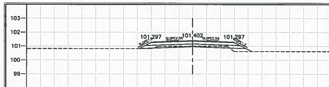
STA. 2+525.000 NGL = 100.997
